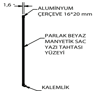
KESİT A-A
